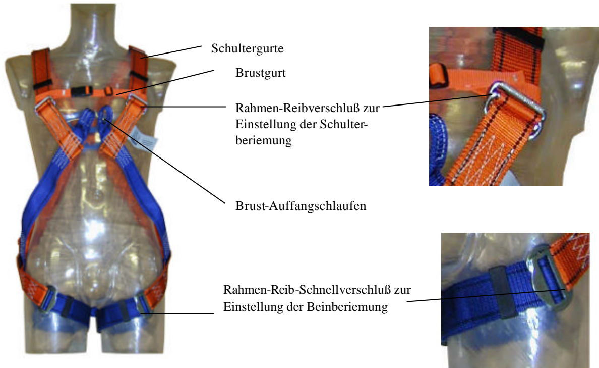
Vorderansicht
