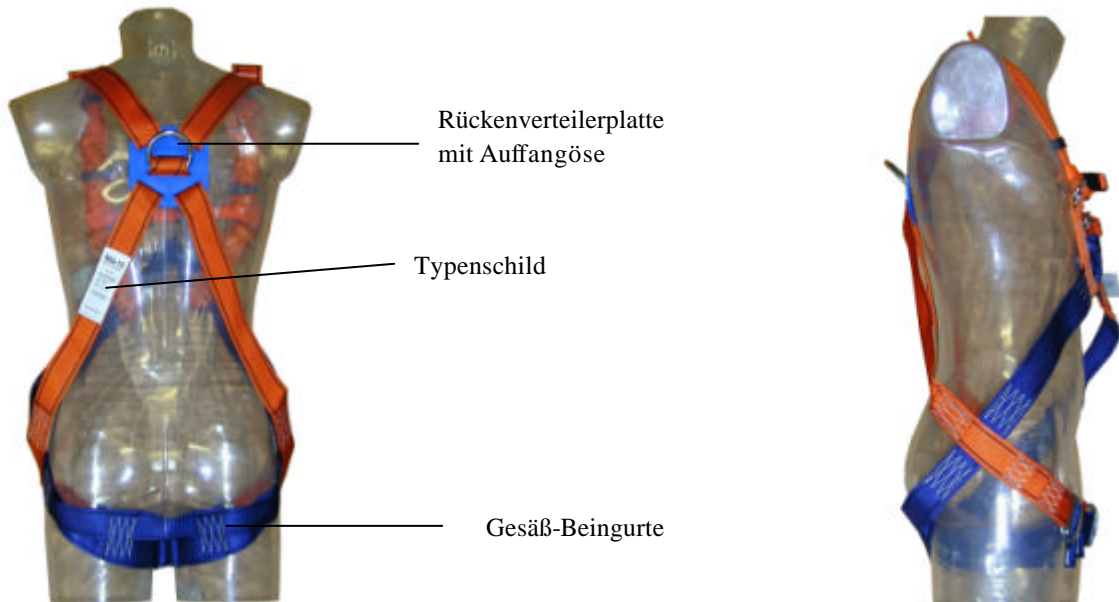
Rückansicht
